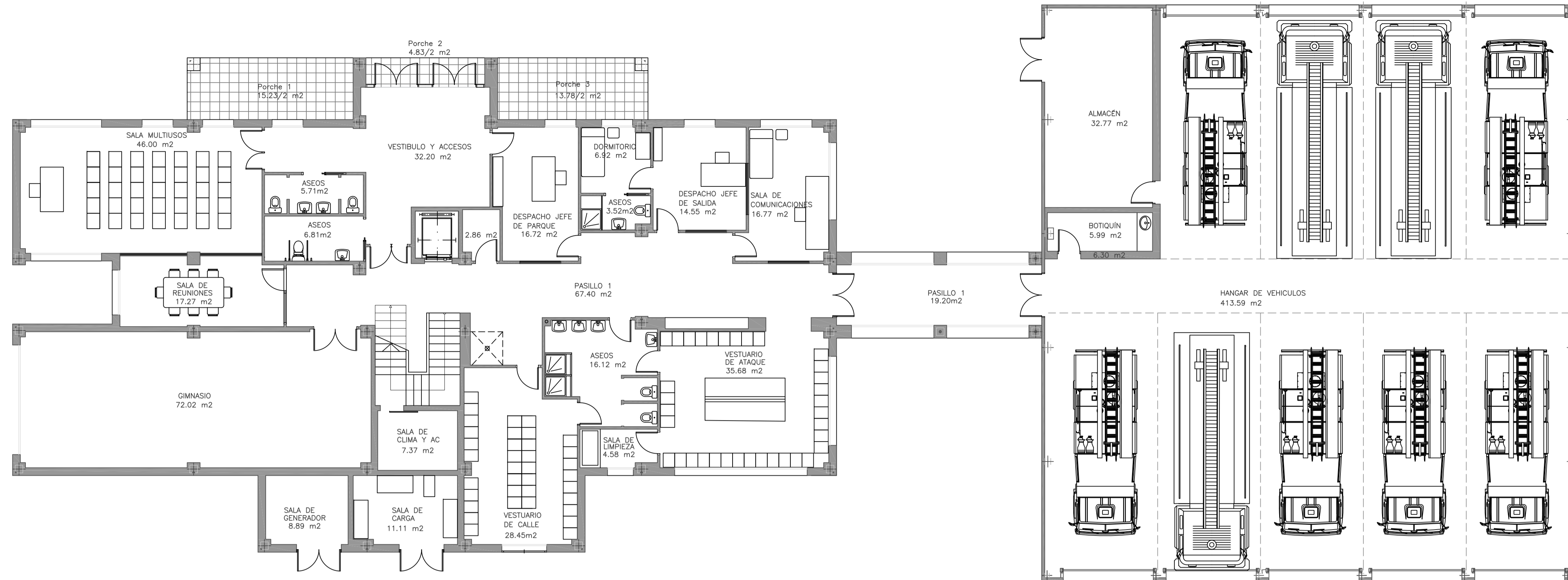
PLANTA BAJA
